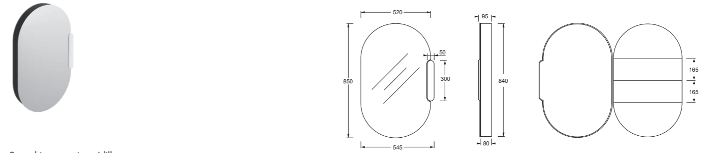
Specchio contenitore Idilla Idilla storage mirror
