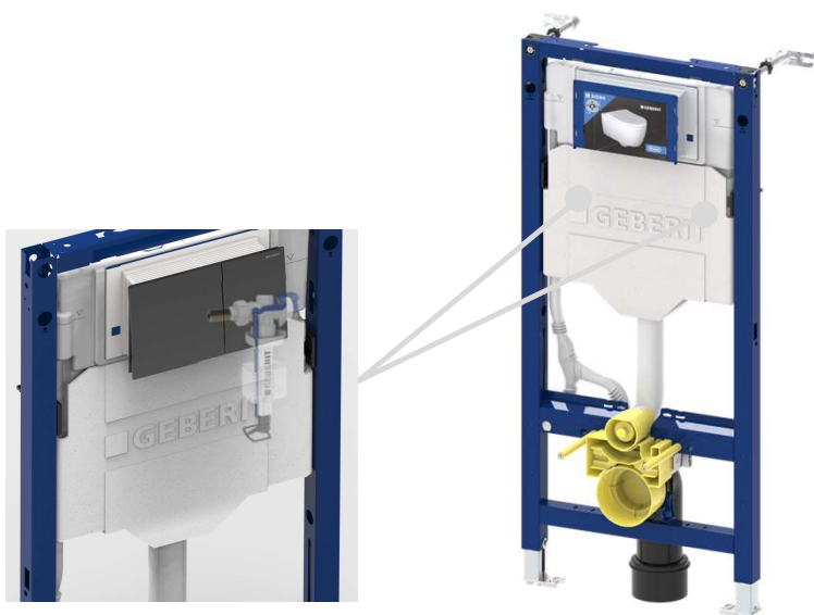
Новая противоконденсатная изоляция
