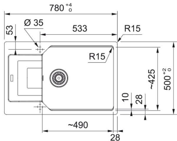
Мойка UBG 611-78, 3 1/2", стоп-вентиль в комплекте, круглый перелив в чаше
